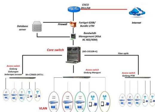
Gambar 5: Perancangan infrastruktur jaringan jangka pendek Fakultas Teknik UNIMA
