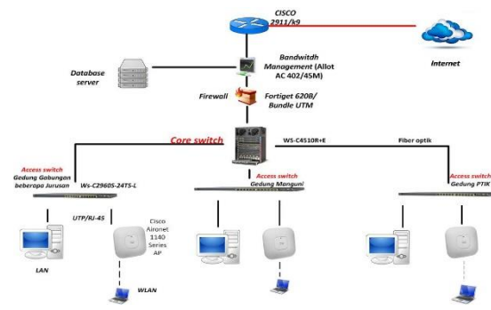
Gambar 4: Skema jaringan yang terimplementasi di Fakultas Teknik UNIMA
