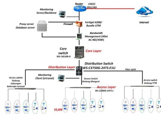
Gambar 6: Perancangan infrastruktur keamanan jaringan Fakultas Teknik UNIMA
